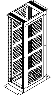
52 mm ölçüde bal peteği havalandırmalı yan panel
