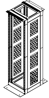
52 mm ölçüde bal peteği havalandırmalı yan panel
