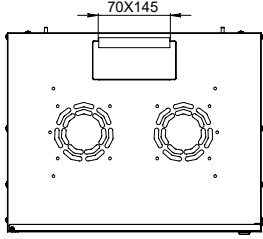
ÜST GÖRÜNÜŞ
