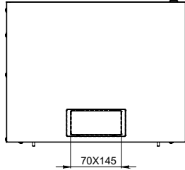
ALT GÖRÜNÜŞ
